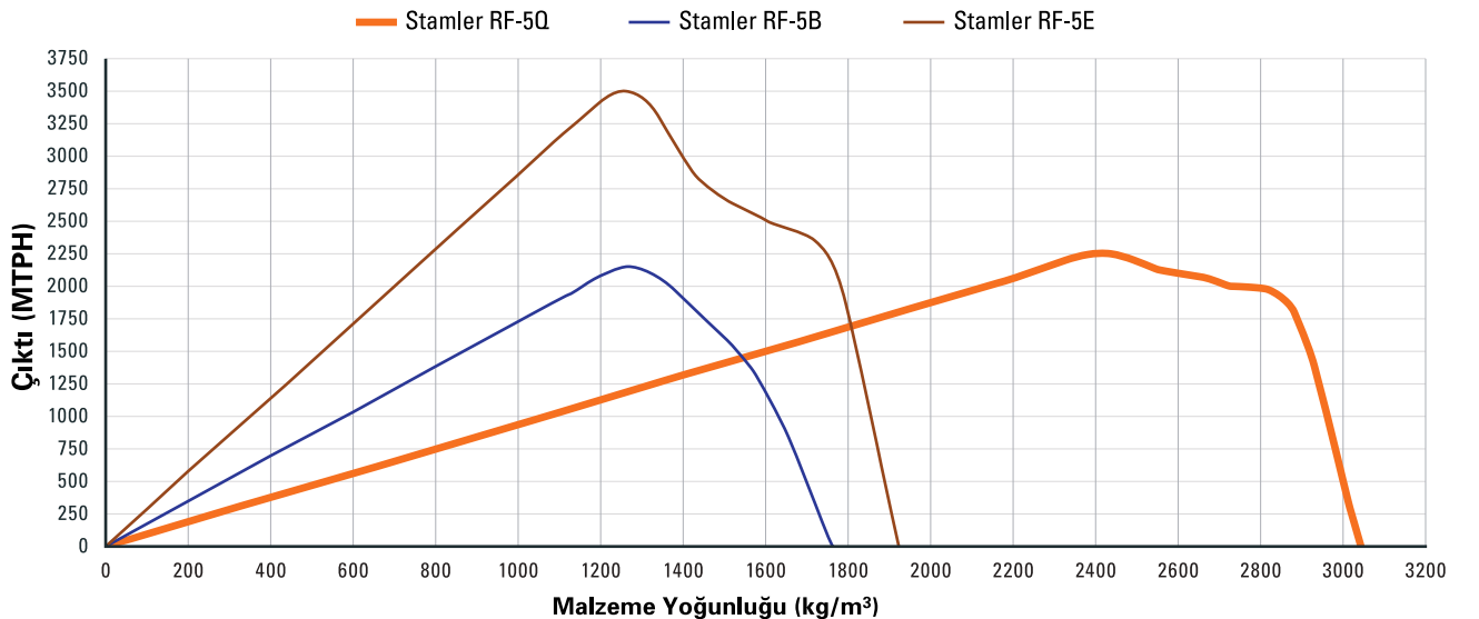
Stamler RF-5 çıktı kapasitesi ile malzeme yoğunluğu karşılaştırması - temel
